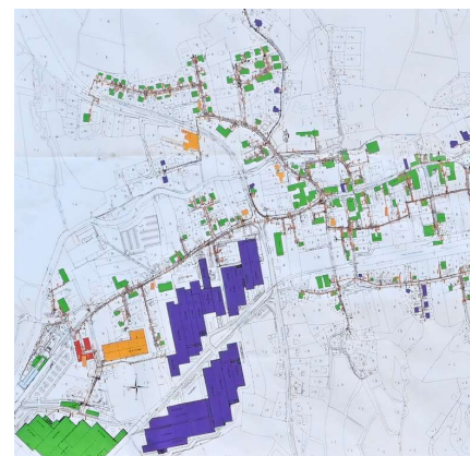
4.000 KW leistet der neue Heizkessel (links). Knapp 16 Kilometer misst das Fernwärme-Leitungsnetz, das mehr als die Hälfte aller Haushalte im Ort erschließt.
