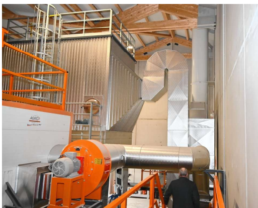
4.000 KW leistet der neue Heizkessel (links). Knapp 16 Kilometer misst das Fernwärme-Leitungsnetz, das mehr als die Hälfte aller Haushalte im Ort erschließt.
