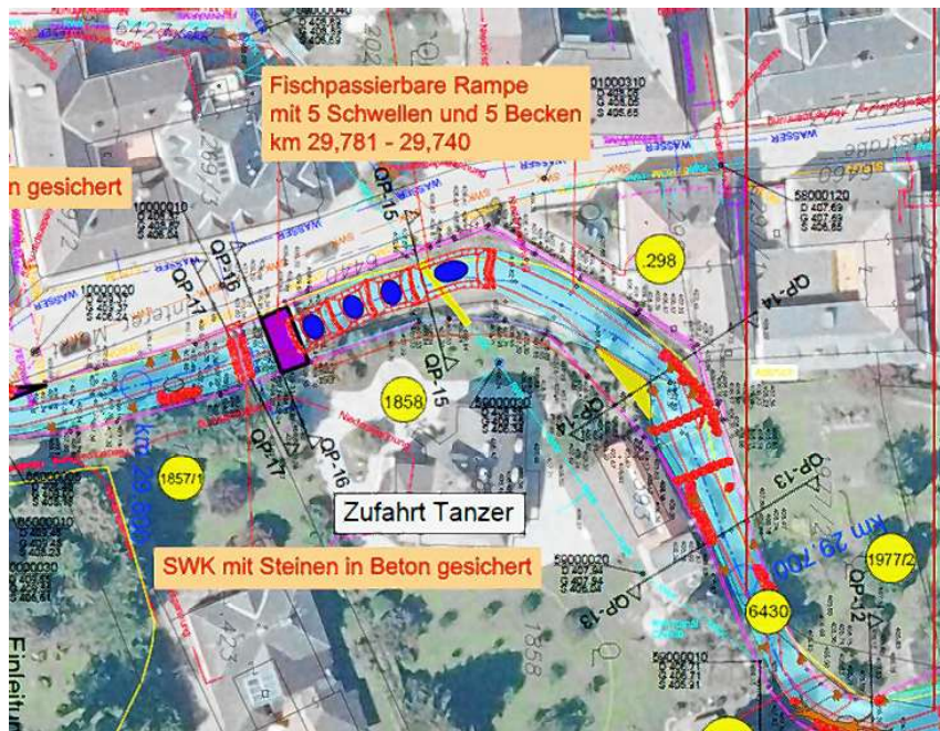
Abtragung Wehranlage Tanzer
